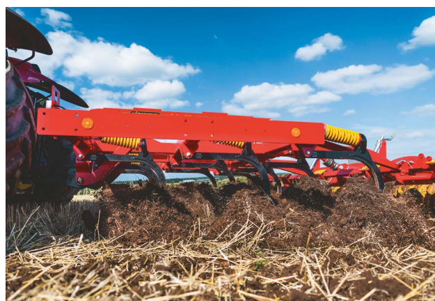
Высокопроизводительные стойки Cultus работают на глубине до 25 см.
